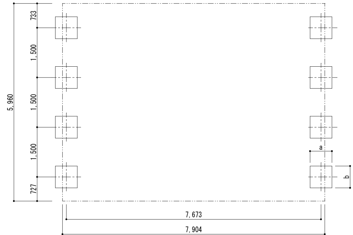
■ 基礎配置図
